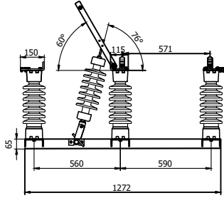
BIÇAK ve TOPRAKLAMA AÇIK GÖRÜNÜŞÜ
