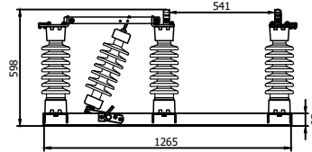
MONTAJI TAMAMLANMIŞ ÜRÜN GÖRÜNTÜSÜ
